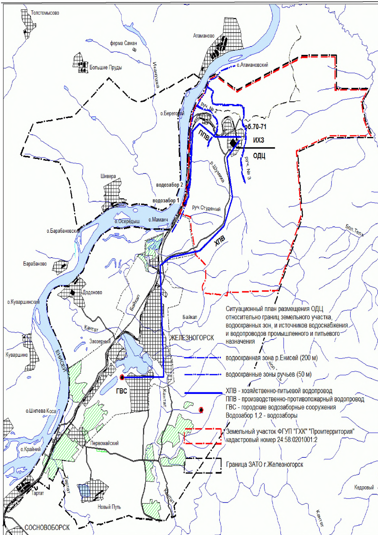
Рисунок 4.3.3.1 – Ситуационный план размещения ОДЦ относительно границ земельного участка ФГУП «ГХК», водоохранных зон, источников водоснабжения и водопроводов промышленного и питьевого водоснабжения.
