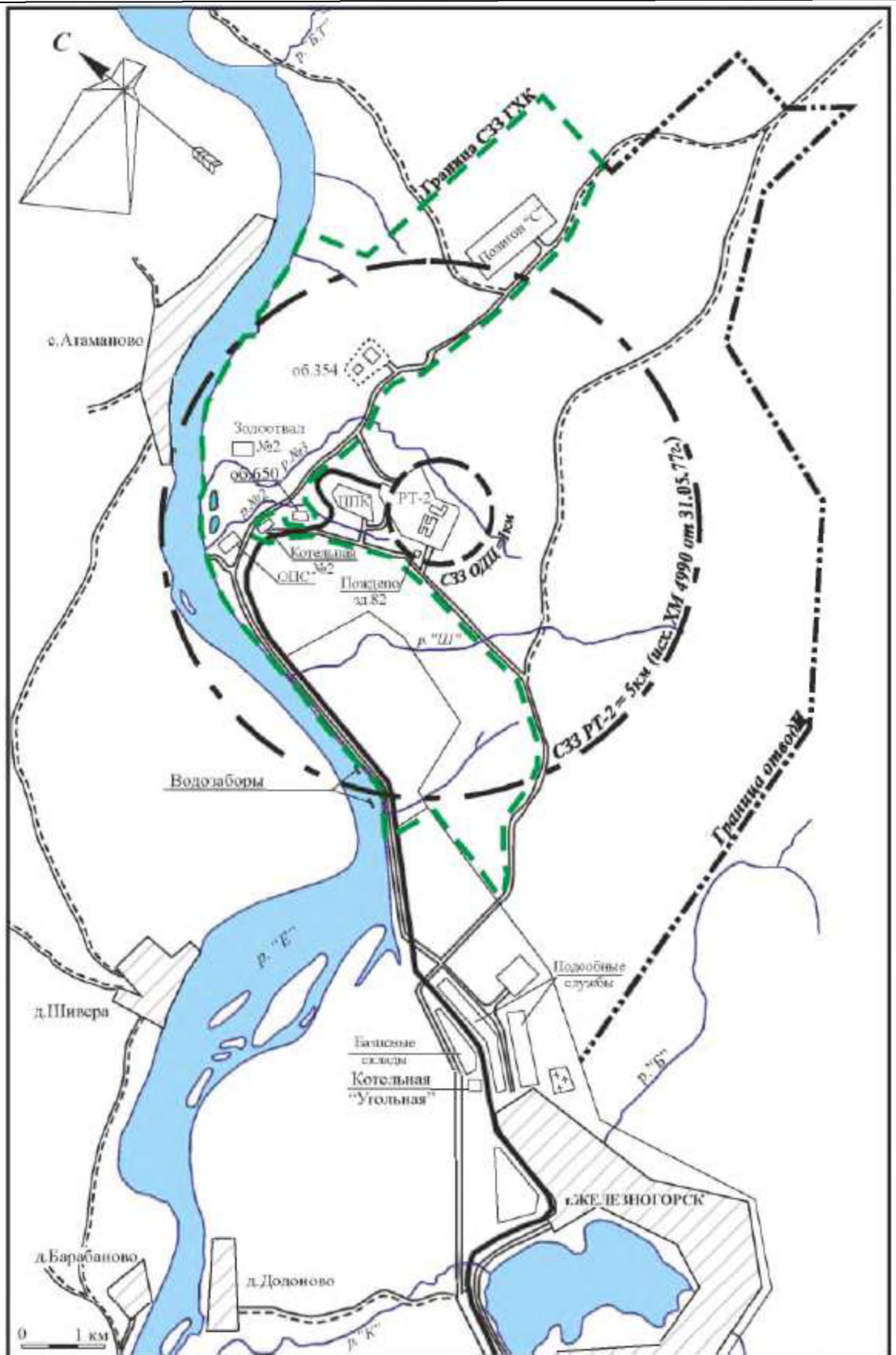
Рисунок 4.3.1.2 – Ситуационный план размещения ОДЦ
