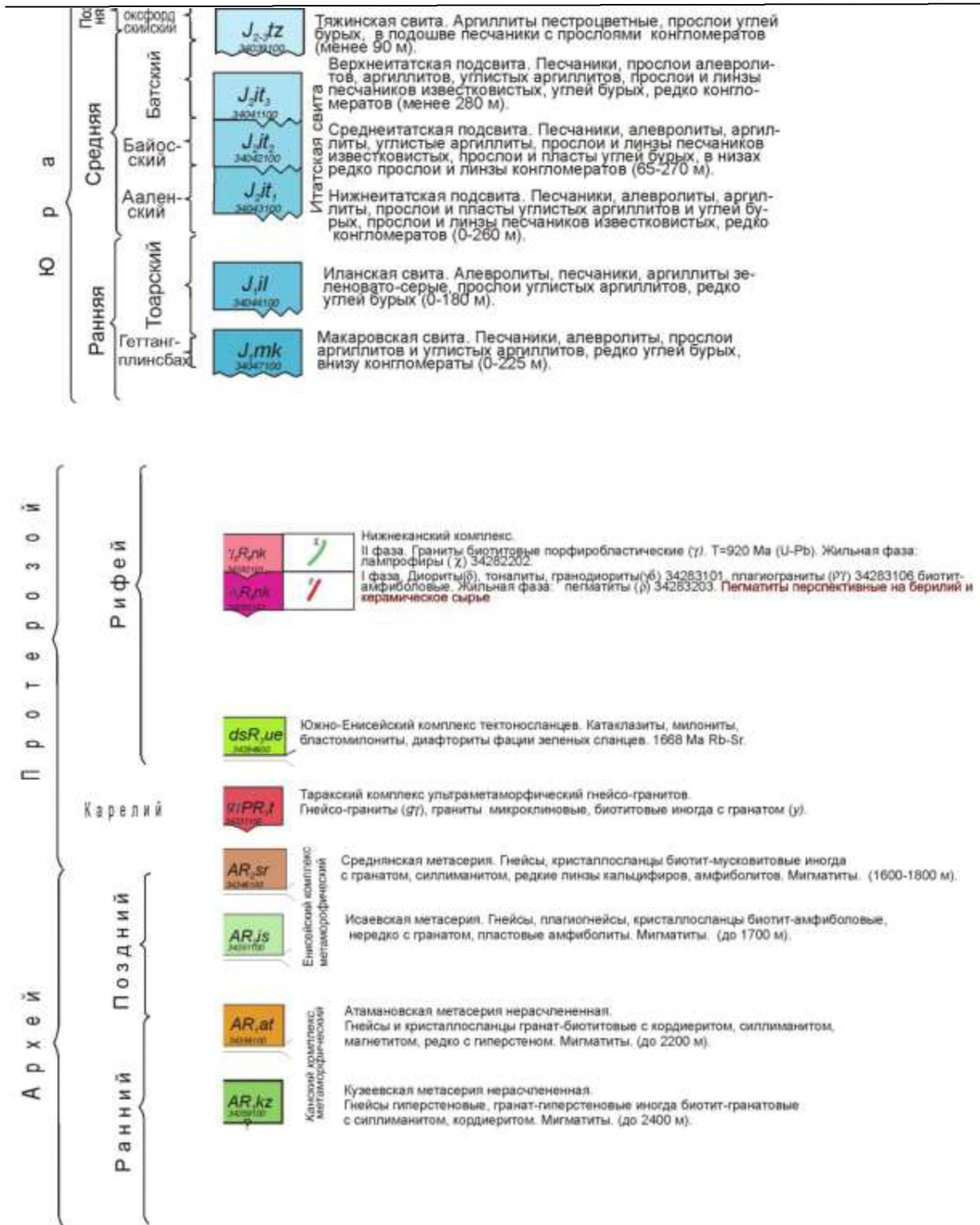
Окончание Рисунка 4.3.5.1.1 – Геологическая карта района Окончание условных обозначений
