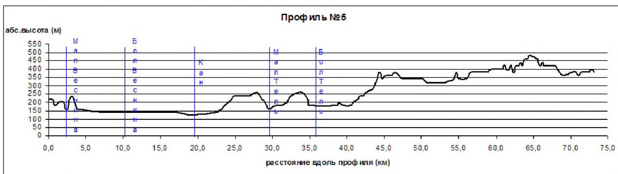
Рисунок 4.3.7.1.7 – Гипсометрический профиль вдоль меридиана 93°51' от р. М.Веснина до верховьев р. Бол. Итат вкрест простирания диагональных и субширотных разломов
