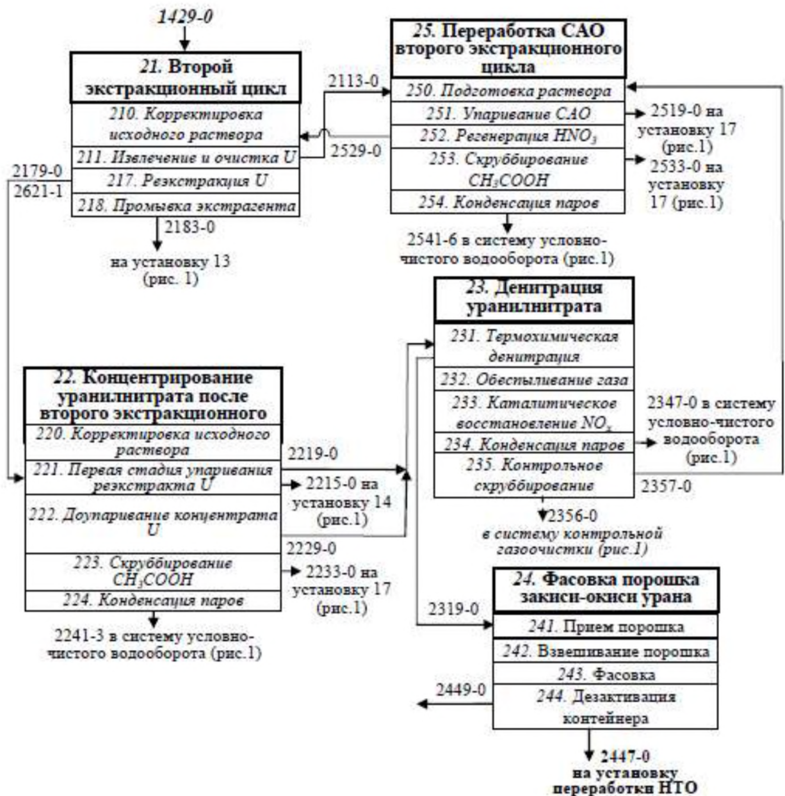
Рисунок 2.3.2 - Блок-схема установок переработки ОЯТ на ОДЦ «ГХК» и связей между ними (второй экстракционный цикл)
