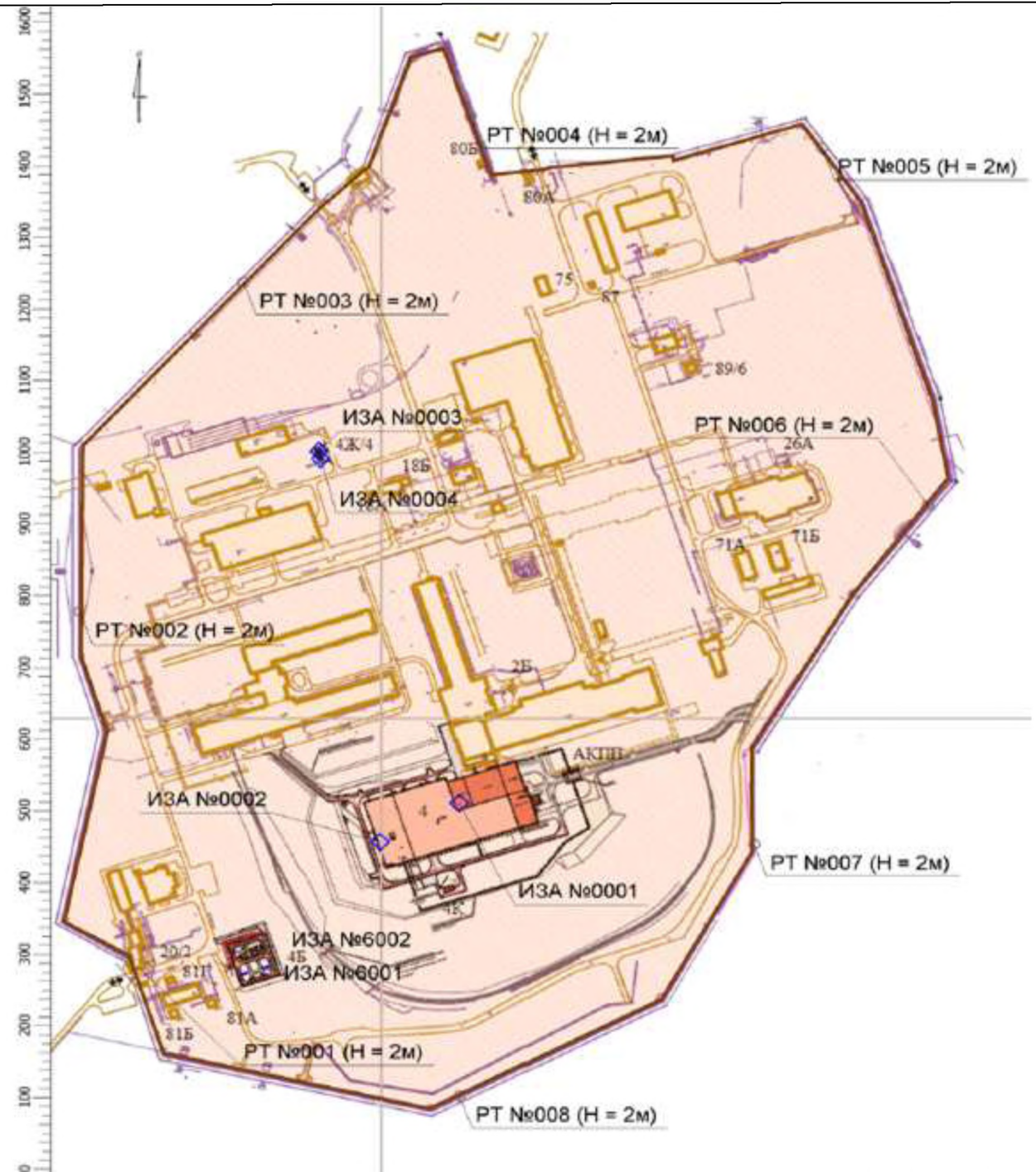
Рисунок 4.4.1.2 – Ситуационный план-схема размещения зданий и источников выбросов загрязняющих веществ при эксплуатации ОДЦ
