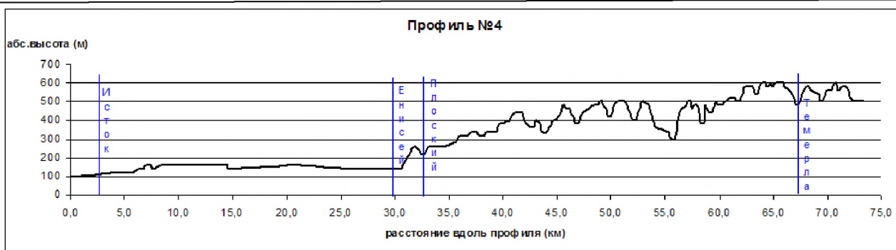
Рисунок 4.3.7.1.6 – Гипсометрический профиль вдоль меридиана 93°39' от р. Исток до р. Темерла вкрест простирания диагональных и субширотных разломов
