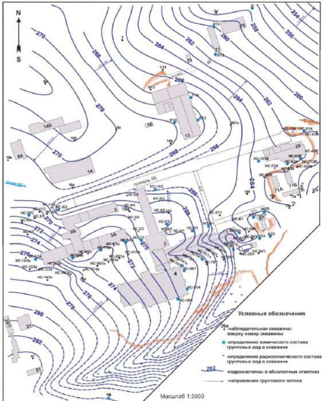
Рисунок 4.8.5.1 - Схема пунктов химического и радиохимического контроля состояния подземных вод на промышленной площадке ЗРТ.
