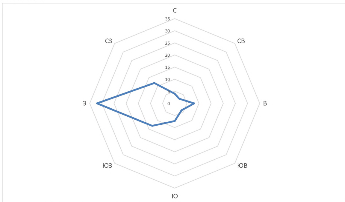
Рисунок 4.3.2.1 - Роза ветров
